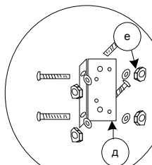
Сборка (Z)
